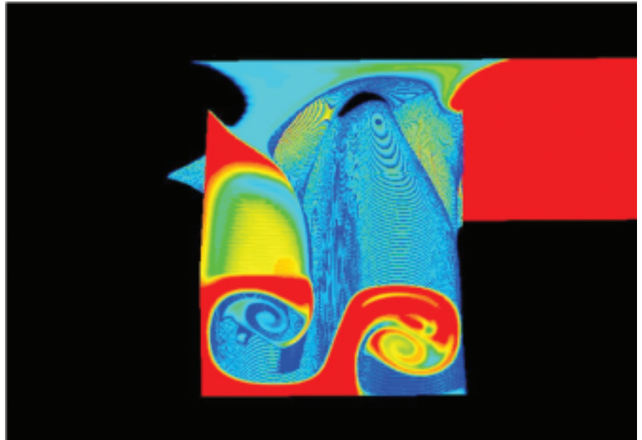
Vermischung eines roten und eines schwarzen Fluids im T-Mikroreaktor (Querschnittfläche 200 \mu\text{m} x 100 \mu\text{m} ). Visualisierung der laminaren Strömungsprofile.
